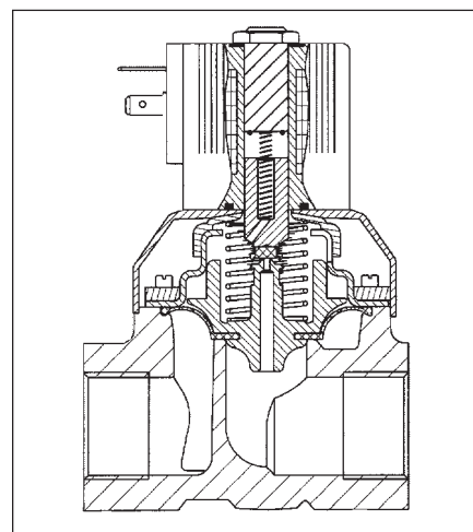
Způsob činnosti 2/2 cestného magnetického ventilu
