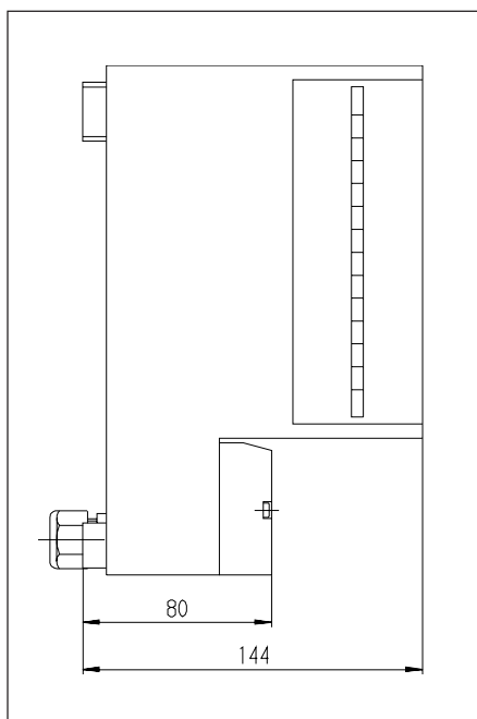
Skříňka monitoru
